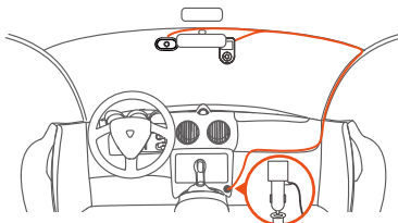
Installation de la lentille DMS et diagramme de câblage
